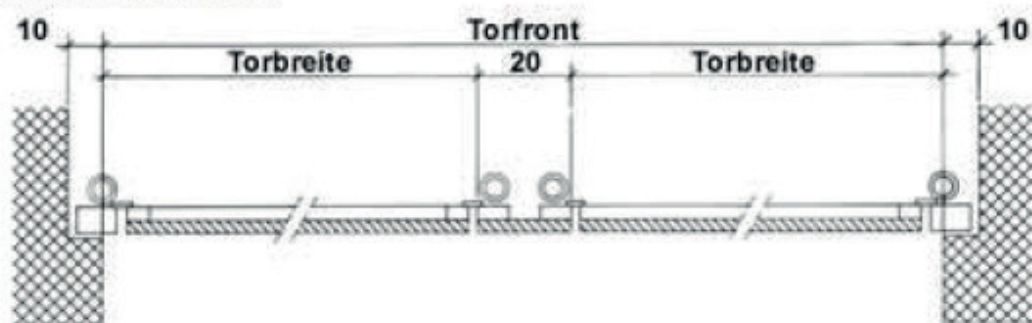
Torfront mit Mittelblende
