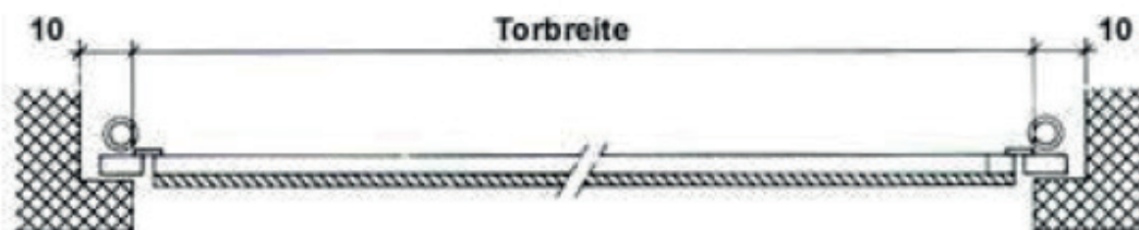
Toreinbau mit seitlichem Anschlag
