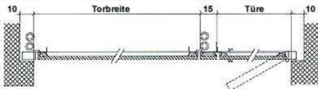
Torfront mit eingebauter Service-Türe (links oder rechts)
