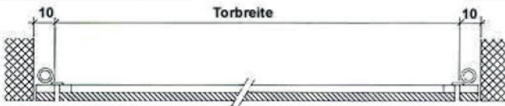
Torfront ohne seitlichem Anschlag
