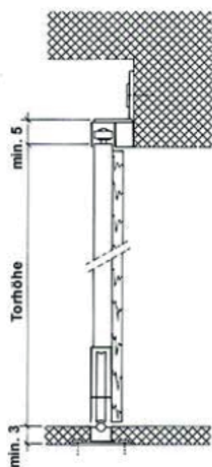
Sturz Detail
